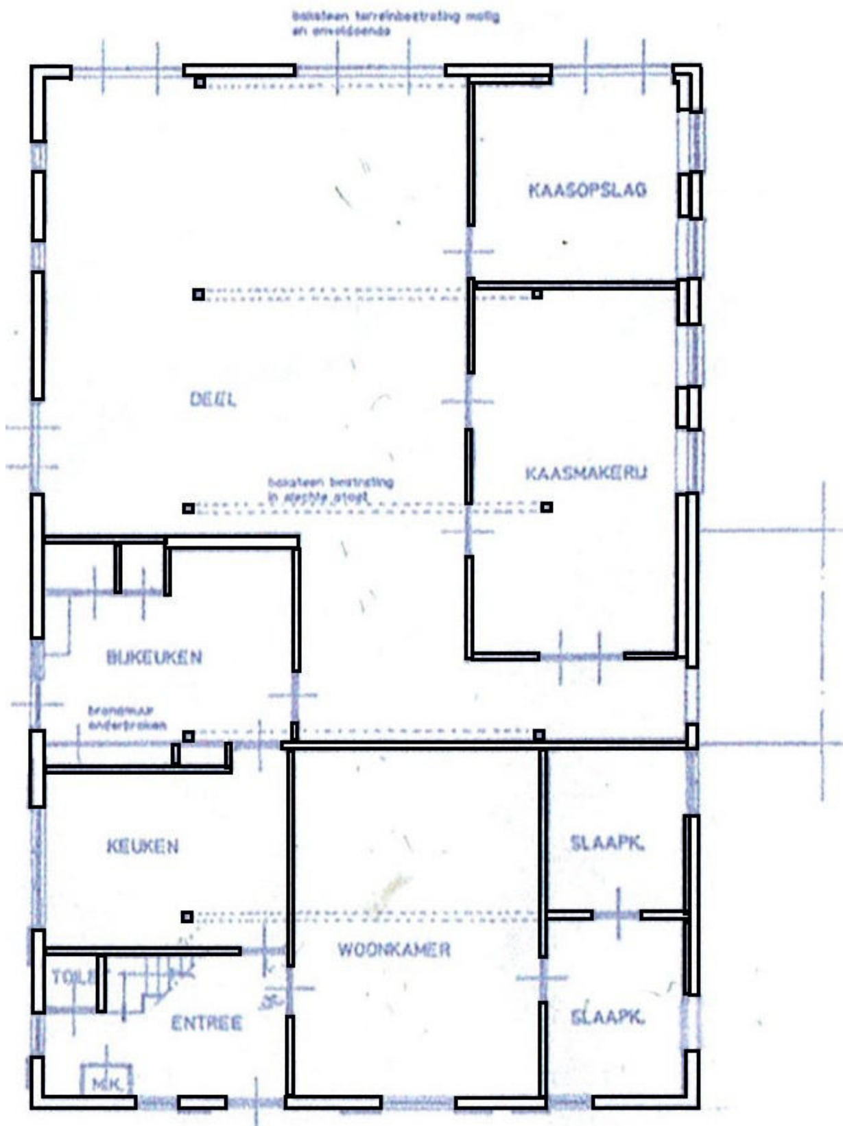
BEGANE GROND
