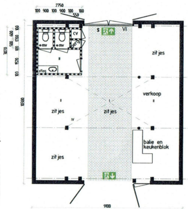
Plattegrond 2023
