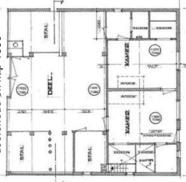
plattegrond 1936
