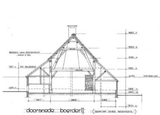
Afwijkende dakhelling vanaf pannen dak door verhogen oostmuur voor 1936
