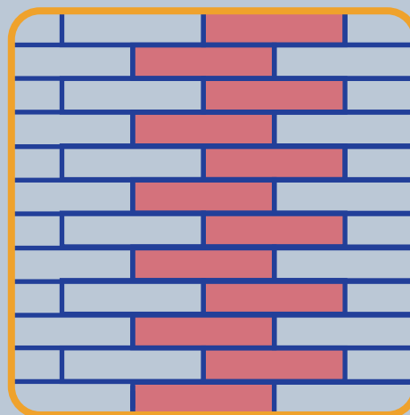
C. HALFSTEENSVERBAND
