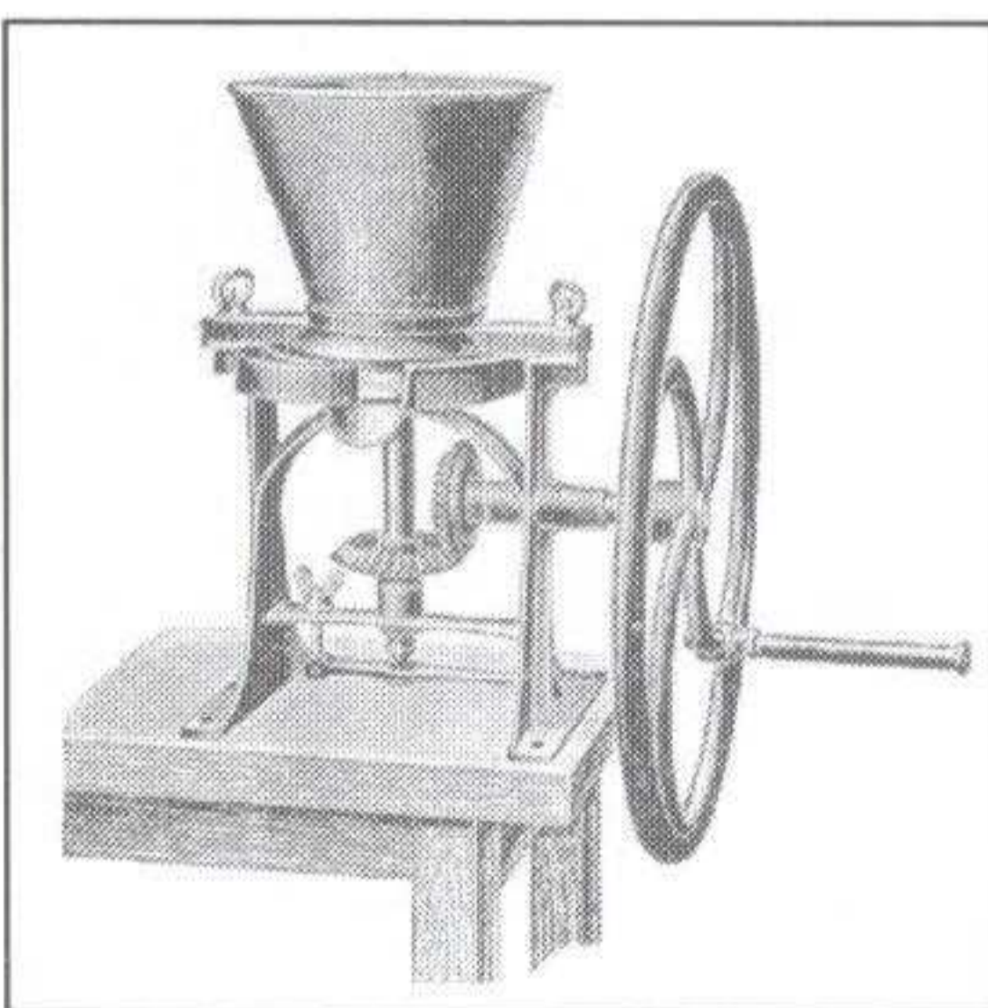
Een conus- of potmolen voor het vermalen van kleurstoffen met lijnolie uit omstreeks 1910
