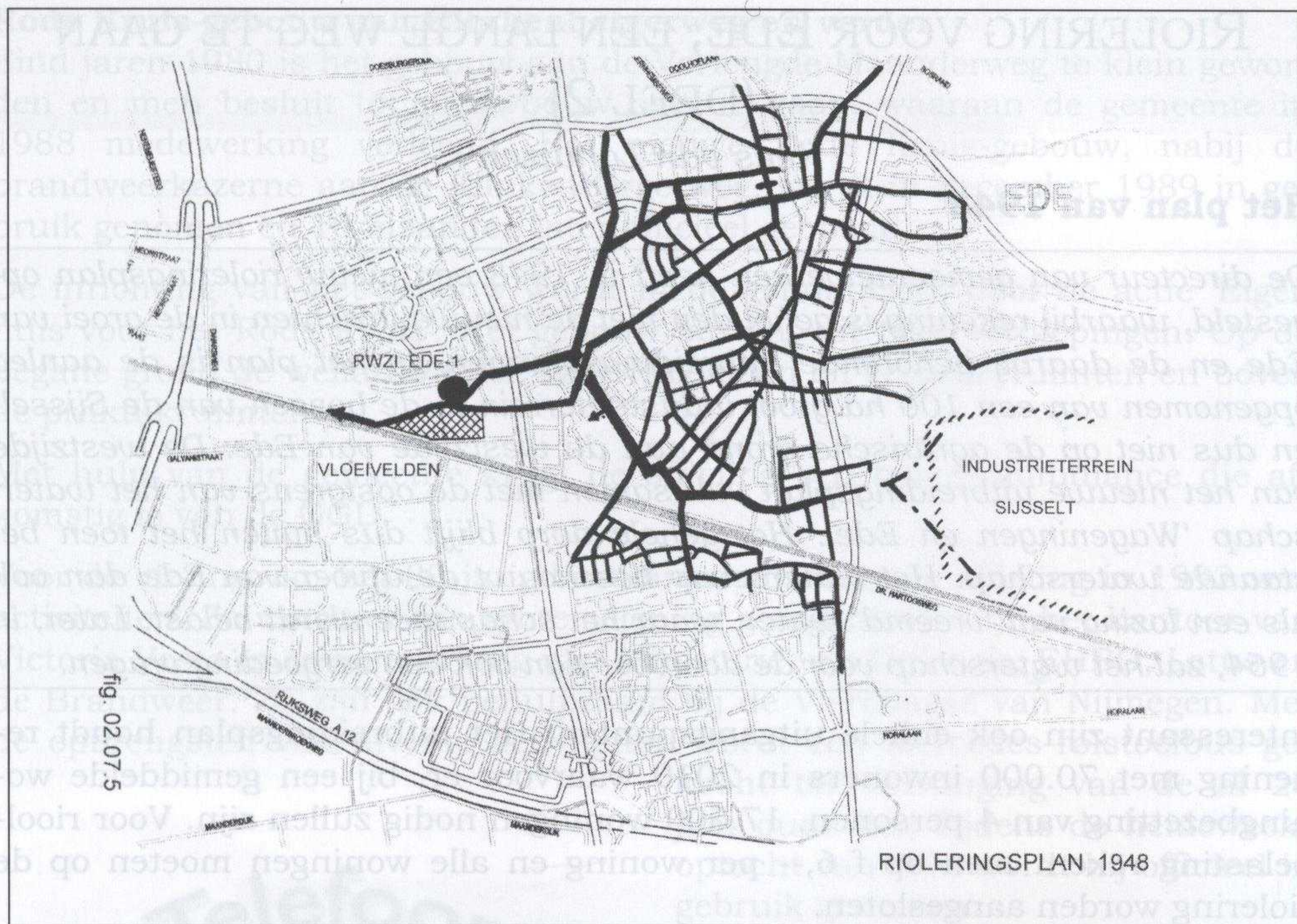
Op deze tekening zijn de hoofdriolen aangegeven op een ondergrond van het huidige Ede.
