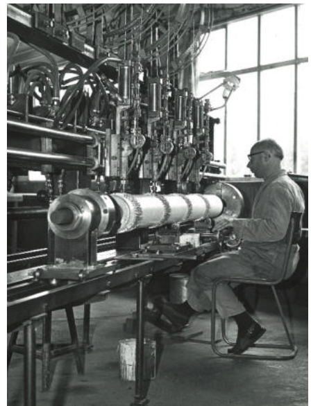
Geautomatiseerd graveren
